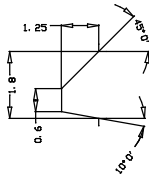
PERFIL DO FILETE ESCALA 10: 1
