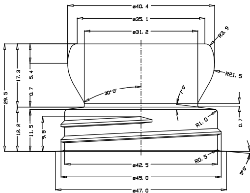
DETALHE DO GARGALO ESCALA 2: 1
